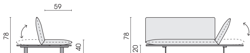
Seitenansicht
